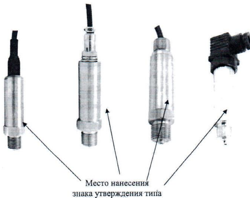
Рисунок 1 – Общий вид датчиков давления класса «малогабаритные»
