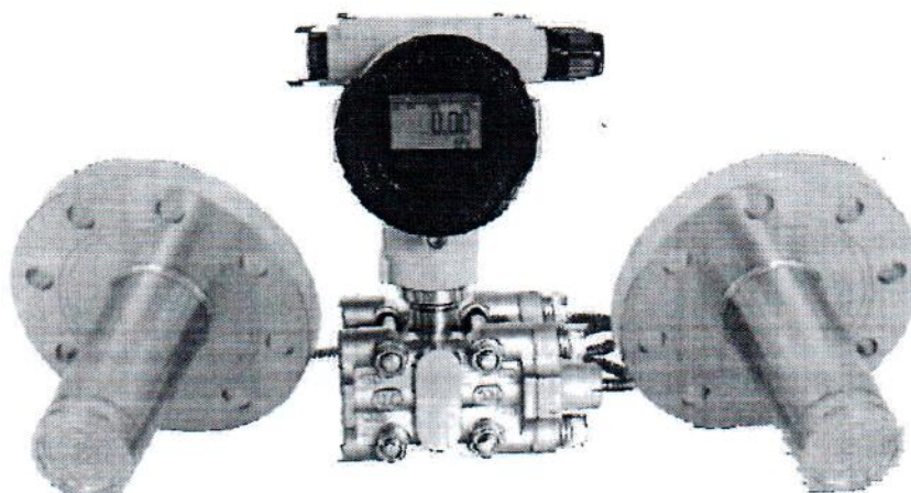
Рисунок 4 – Общий вид датчиков давления класса «премиум»
