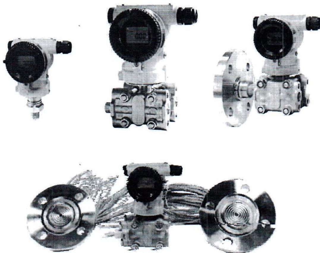
Рисунок 3 – Общий вид датчиков давления класса «премиум»
