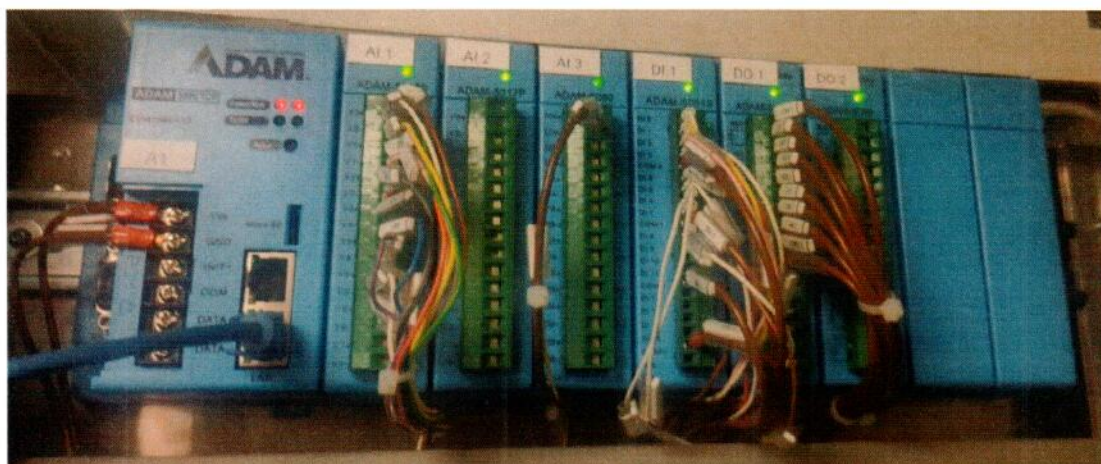
а) программируемый контроллер ADAM-5000 с измерительными модулями из состава системы
