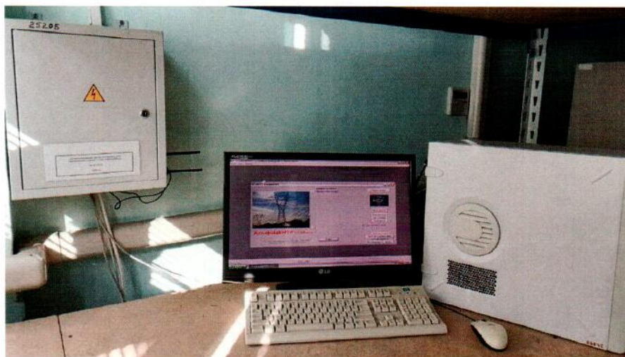
а) автоматизированное рабочее место пользователей (АРМ) АСКУЭ
