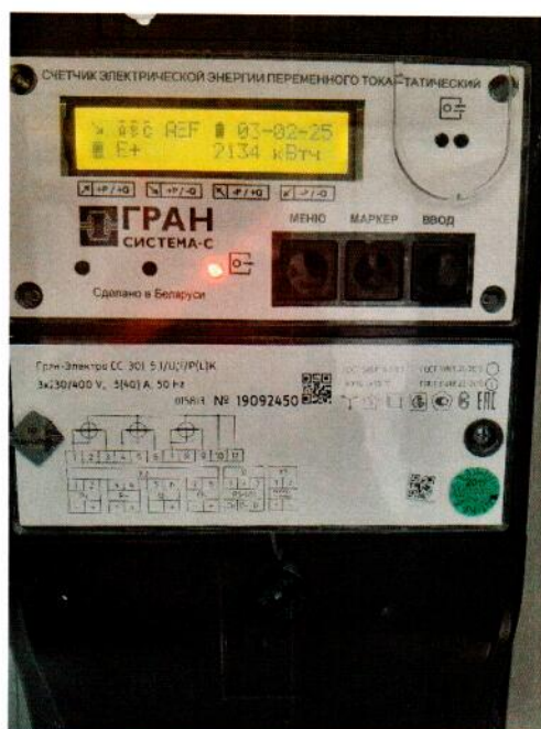
Измерительный канал № 3
