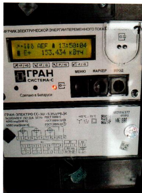
Измерительный канал № 2
