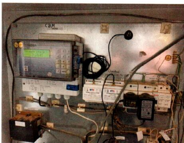
а) шкаф учёта АСКУЭ
