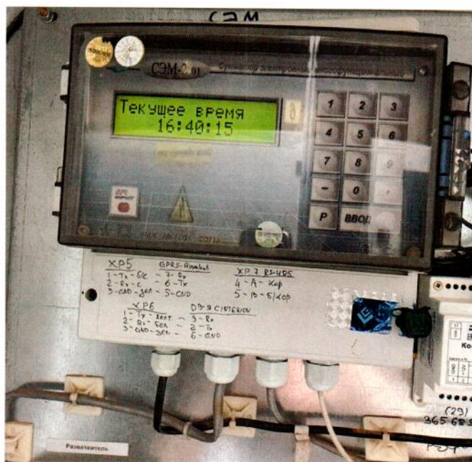
б) сумматор в шкафу учёта АСКУЭ
