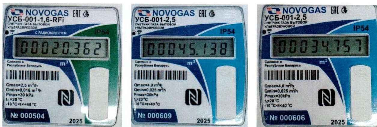
Рисунок 1.2 – Фотография маркировки счетчиков газа бытовых ультразвуковых УСБ-001 (изображение носит иллюстративный характер)
