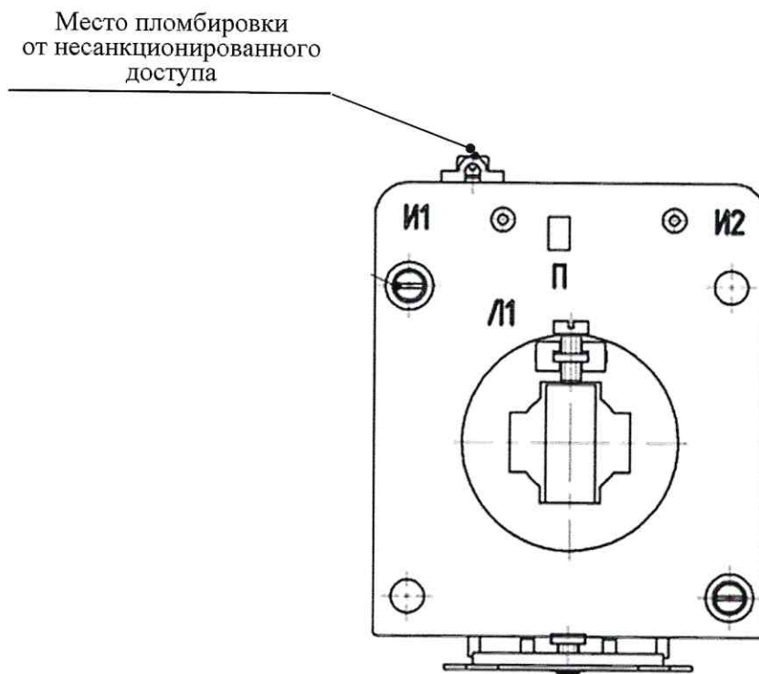
Рисунок 3.1 – Схема пломбировки от несанкционированного доступа трансформаторов тока ТОП-Н-0,66
