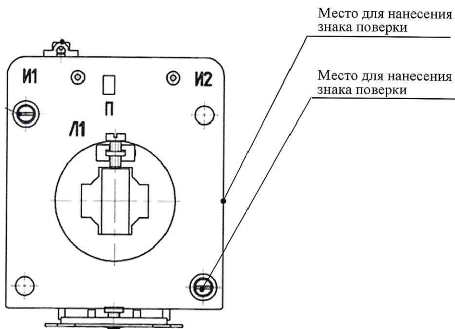
Рисунок 2.2 – Схема (рисунок) с указанием места для нанесения знака поверки средств измерений трансформаторов тока ТШП-Н-0,66
