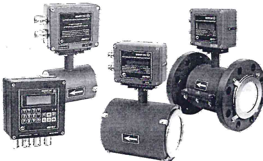
Рисунок 1 – Общий вид расходомеров-счетчиков электромагнитных «ВЗЛЕТ ЭМ»
