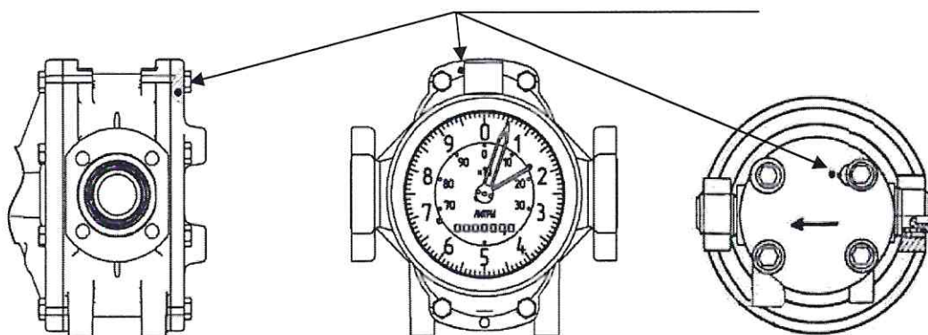
Рисунок 12 – Схемы пломбировки ППО
