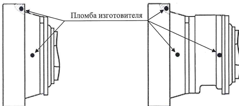
Рисунок 15 – Схема пломбировки ВП СУ+УСС
