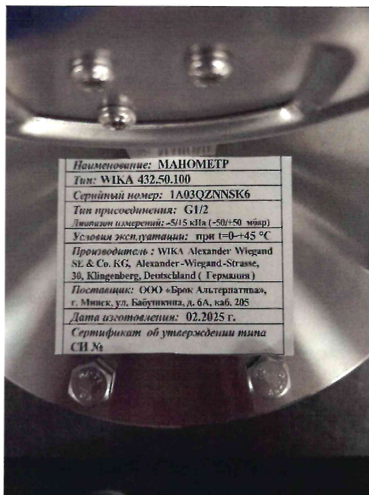
Рисунок 1.1 – Фотография общего вида манометра WIKA 432.50.100 № 1A03QZNNSK6
