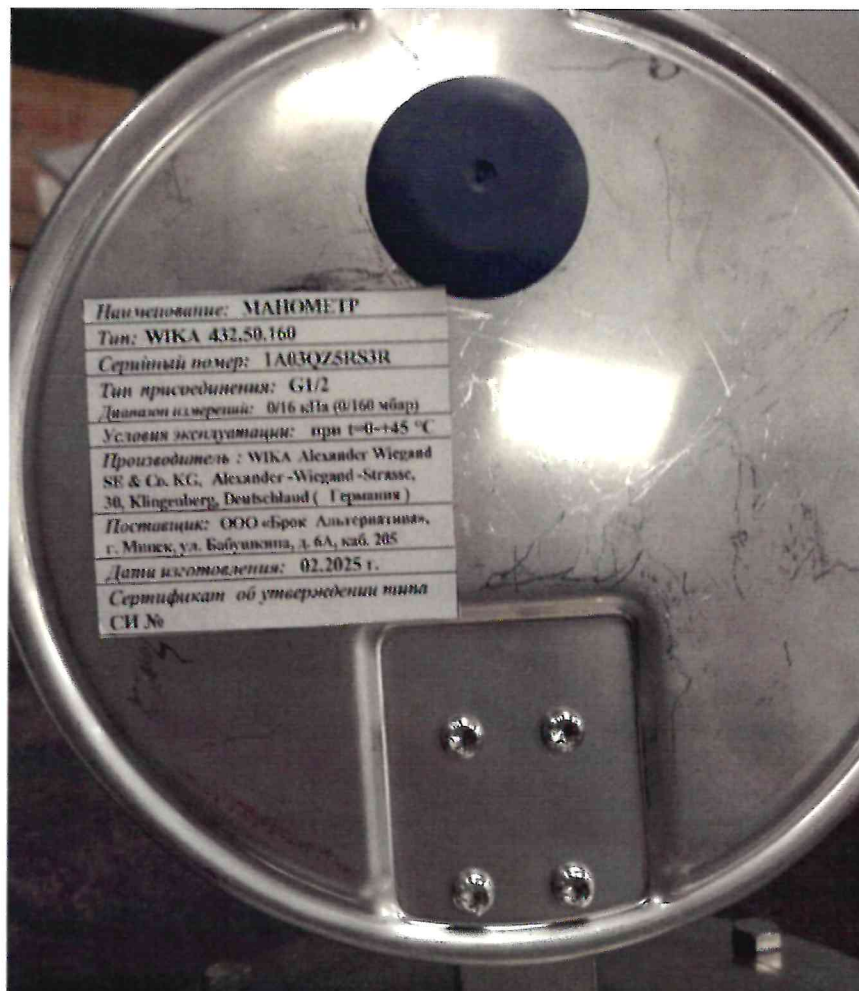
Рисунок 1.2 – Маркировка манометра WIKA 432.50.160 № 1A03QZ5RS3R
