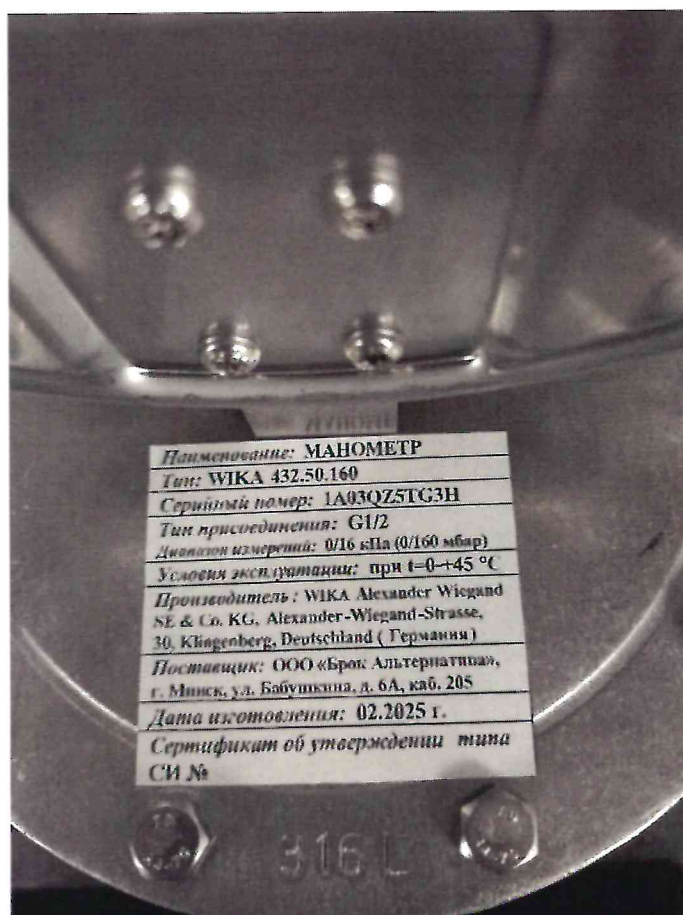
Рисунок 1.2 – Маркировка манометра WIKAI 432.50.160 № 1A03QZ5TG3H
