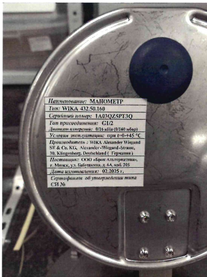
Рисунок 1.2 – Маркировка манометра WIKА 432.50.160 № 1А03QZ5PT3Q
