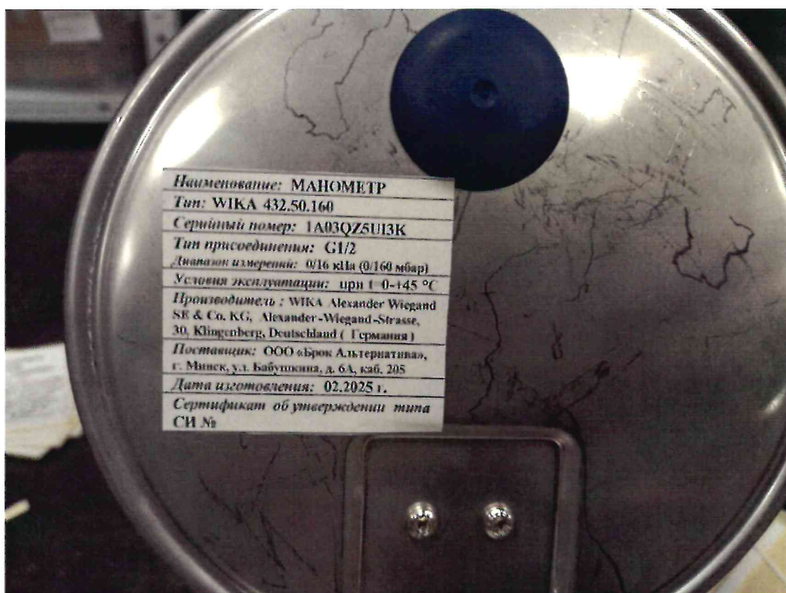
Рисунок 1.2 – Маркировка манометра WIKА 432.50.160 № 1А03QZ5UI3К
