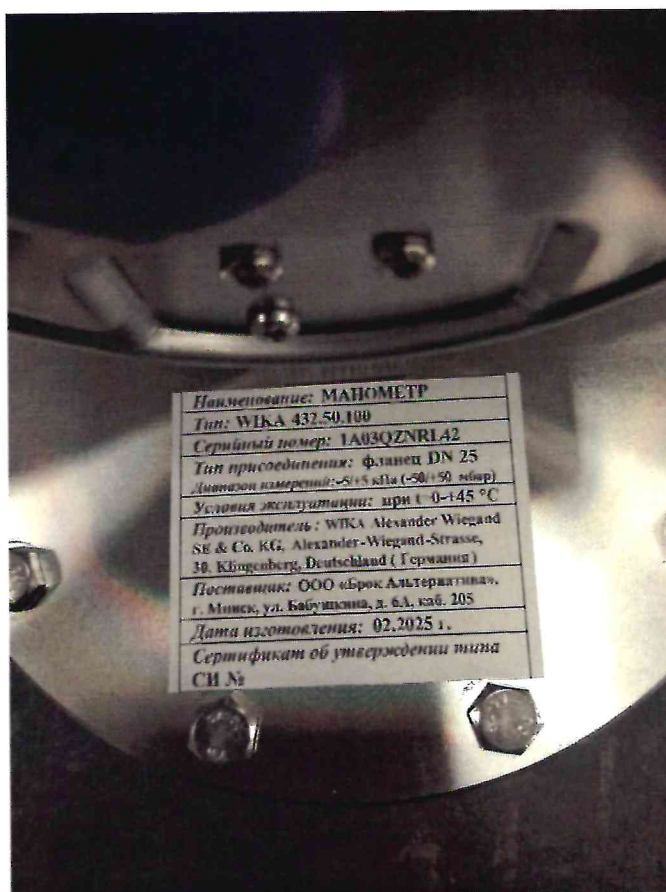
Рисунок 1.1 – Фотография общего вида манометра WIKA 432.50.100 № 1A03QZNRL42
