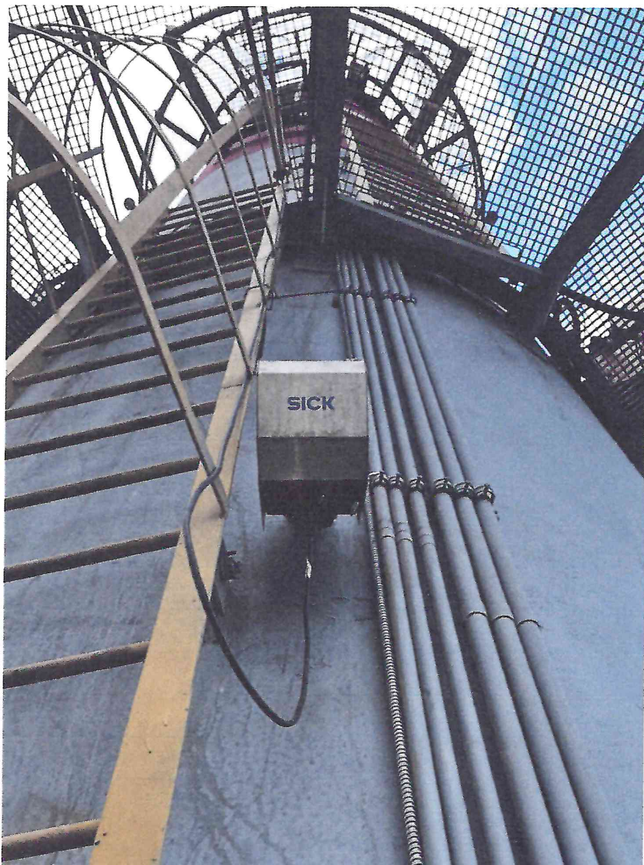
Рисунок 1.3 – Фотография датчиков измерителя скорости газового потока. Система автоматизированная контроля и учета выбросов № СЭ.20322.АСК.001.УХЛ1 от дымовой трубы ДСП 1 ист. выбросов № 0001. ОАО «БМЗ» № СЭ.20322.АСК.001.УХЛ1
