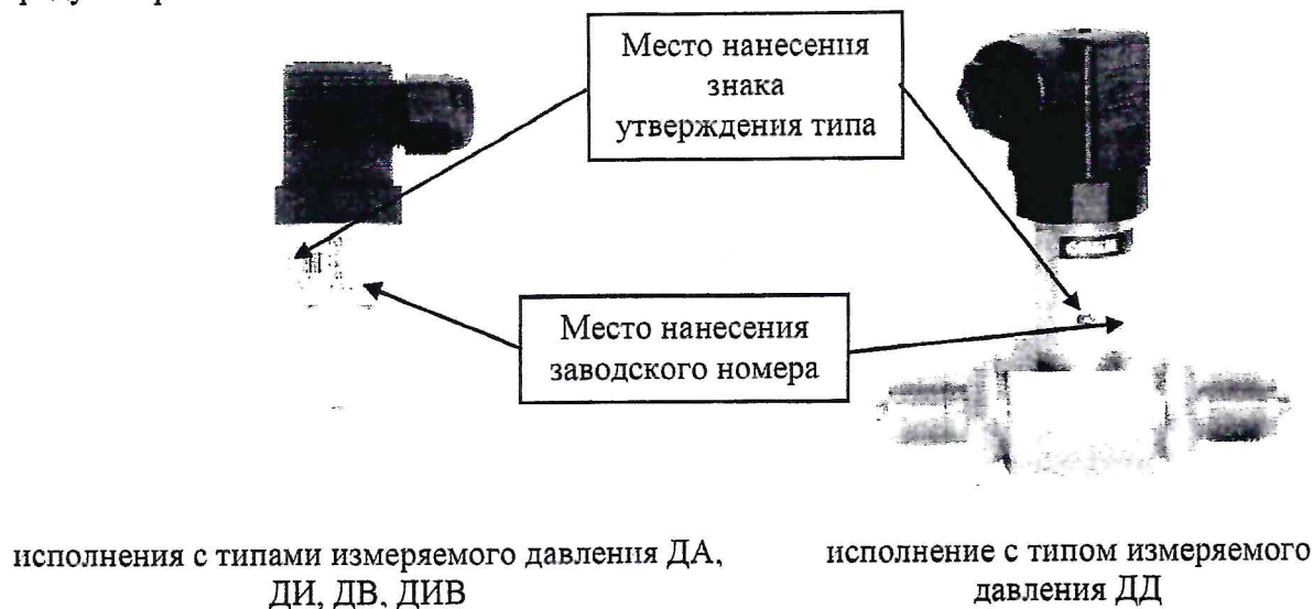
Рисунок 2 – Общий вид преобразователей давления измерительных ОВЕН ПД100И с разъёмом стандарта DIN43650 (EN175301-803) с указанием места нанесения знака утверждения типа, места нанесения заводского номера
