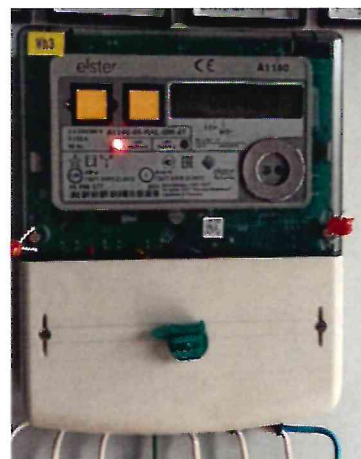
Измерительный канал № 4
