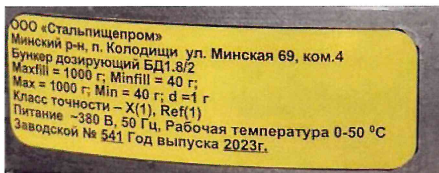
Рисунок 1.2 – Маркировка бункера дозирующего БД1.8/2 № 541
