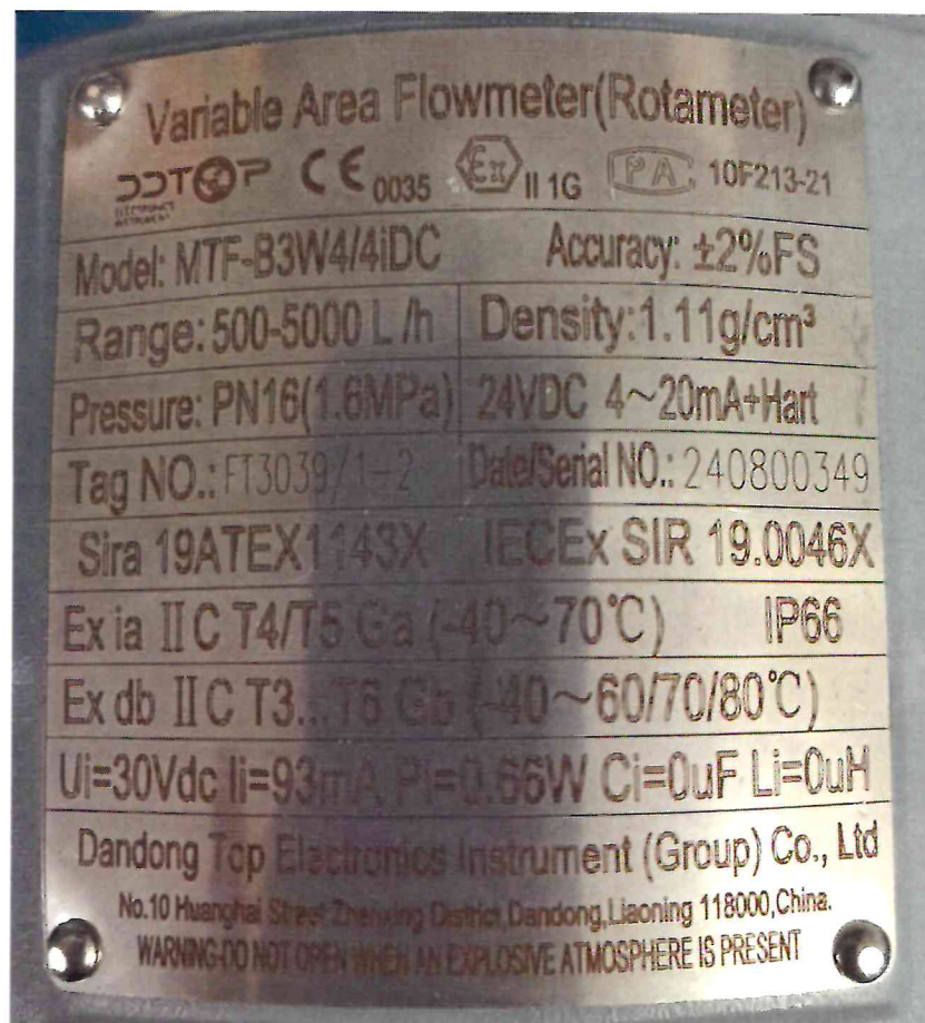
Рисунок 1.2 – Фотография маркировки расходомера поплавкового MTF-B3W4/4iDC № 240800349
