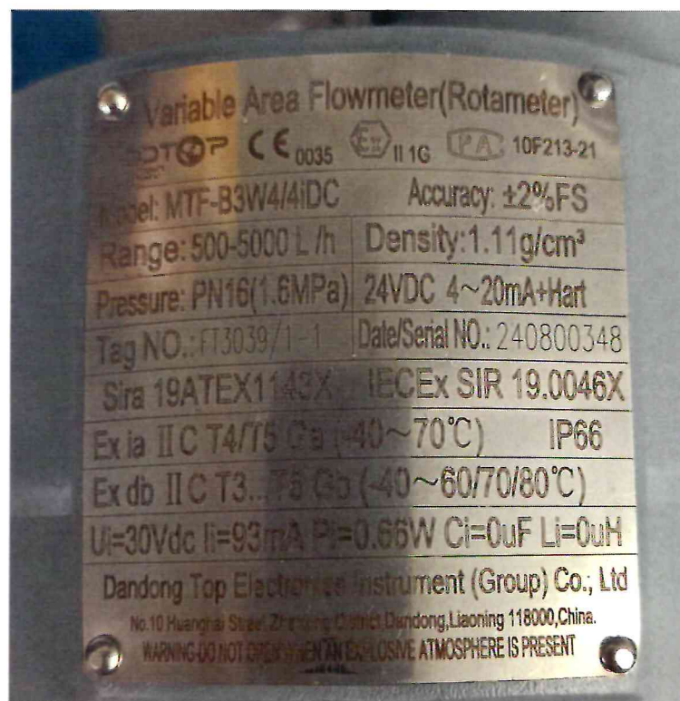
Рисунок 1.2 – Фотография маркировки расходомера поплавкового MTF-B3W4/4iDC № 240800348
