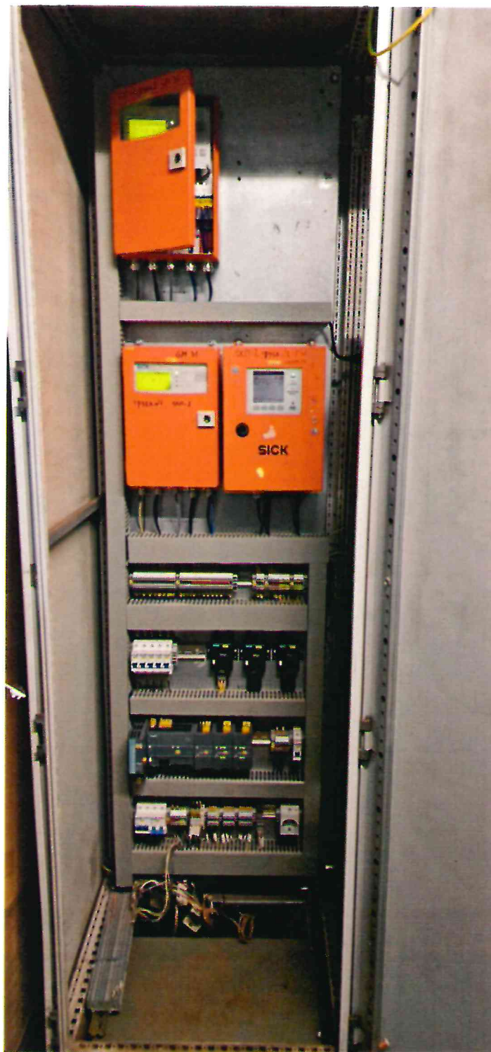
Рисунок 1.1 – Фотография общего вида. Система автоматизированная контроля и учета выбросов № СЭ.20322.АСК.002.УХЛ1 от дымовой трубы ДСП-2 ист. выбросов № 0002. ОАО «БМЗ» № СЭ.20322.АСК.002.УХЛ1
