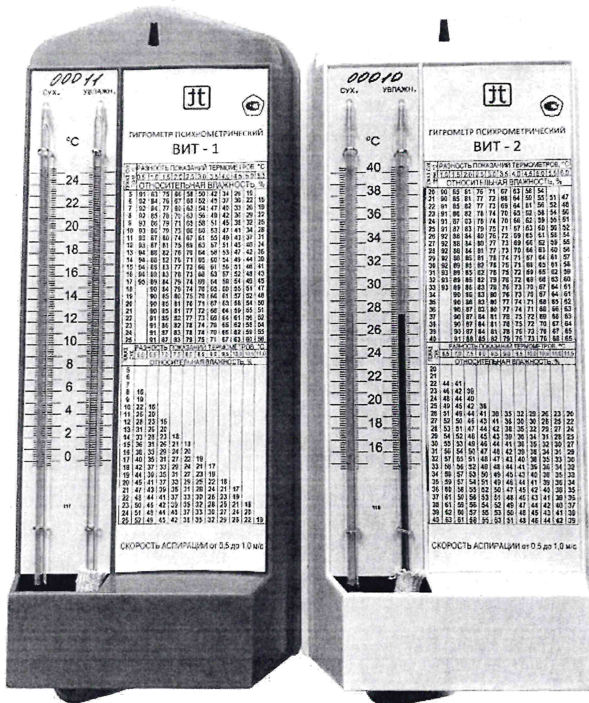
Рисунок 1 – Общий вид гигрометров психрометрических ВИТ-1 и ВИТ-2
