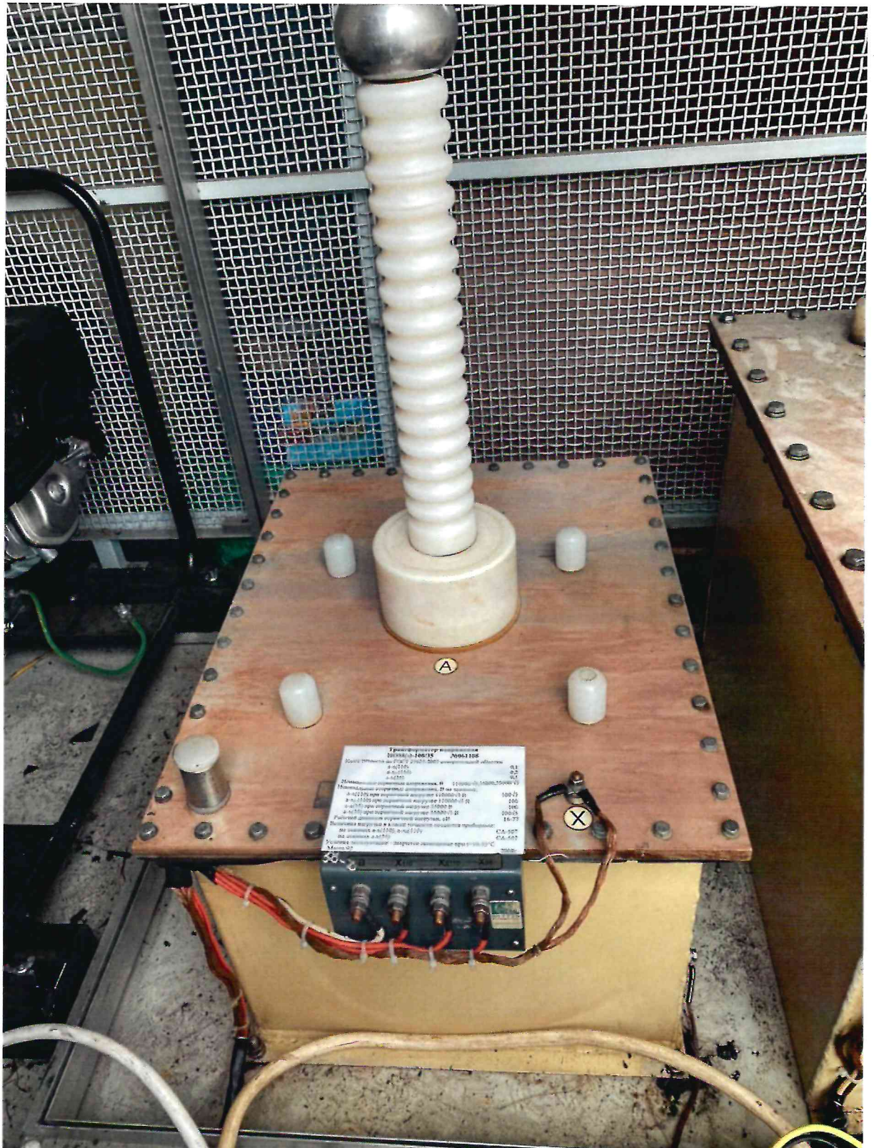
Рисунок 1.1 – Фотография общего вида трансформатора напряжения НОМ(э)-110/35 № 061108
