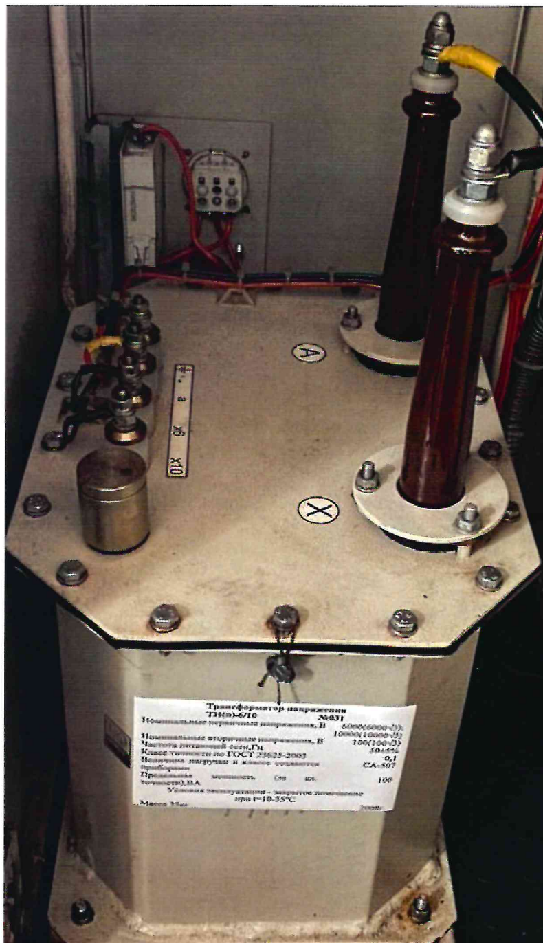
Рисунок 1.1 – Фотография общего вида трансформатора напряжения ТН(п)-6/10 № 031
