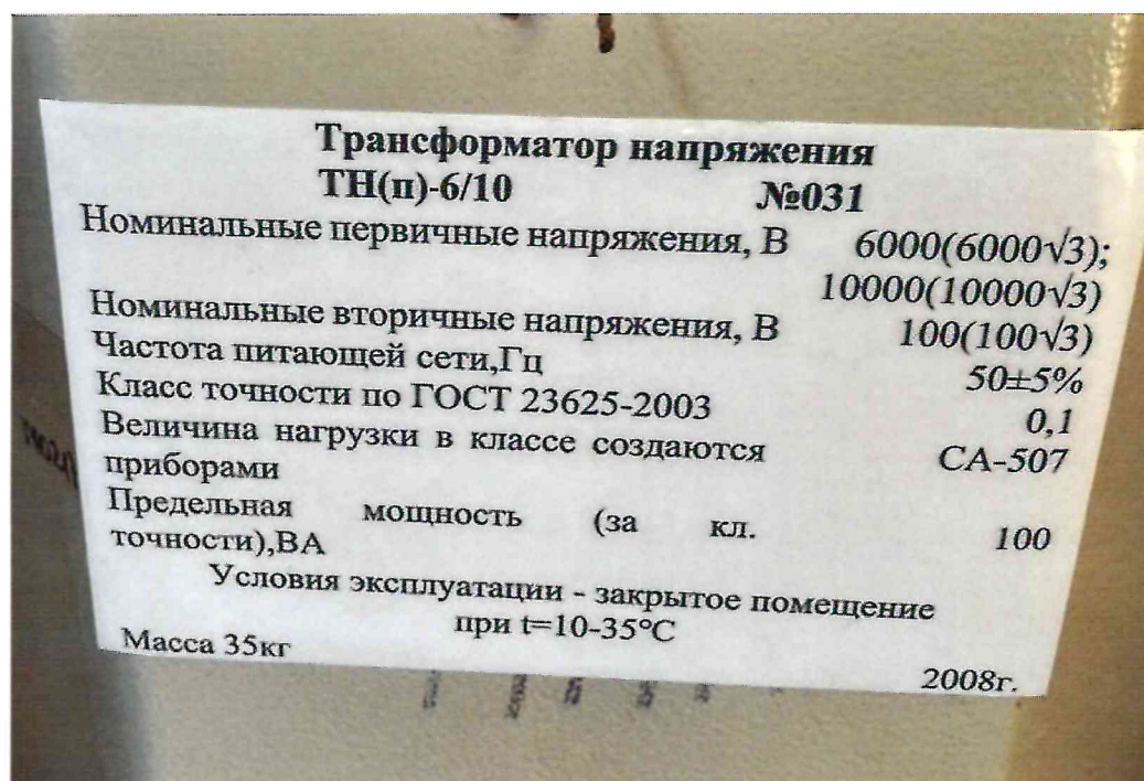
Рисунок 1.2 – Фотография маркировки трансформатора напряжения ТН(п)-6/10 № 031
