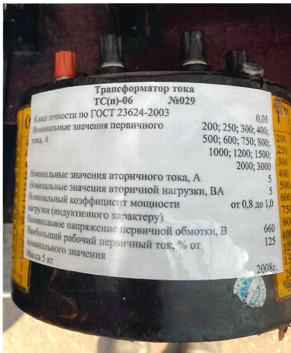
Рисунок 1.2 – Фотография маркировки трансформатора тока ТС(П)-06 № 029
