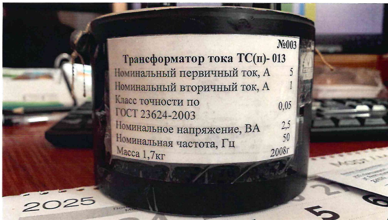
Рисунок 1.2 – Фотография маркировки трансформатора тока ТС(п)-013 № 003
