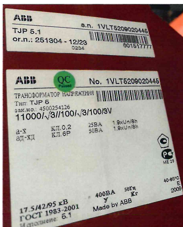
Рисунок 1.2 – Фотография маркировки трансформатора напряжения ТJP 5.1 № 1VLT5209020445
