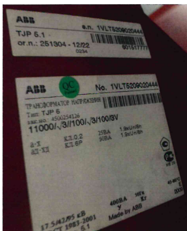
Рисунок 1.2 – Фотография маркировки трансформатора напряжения ТJP 5.1 № 1VLT5209020444
