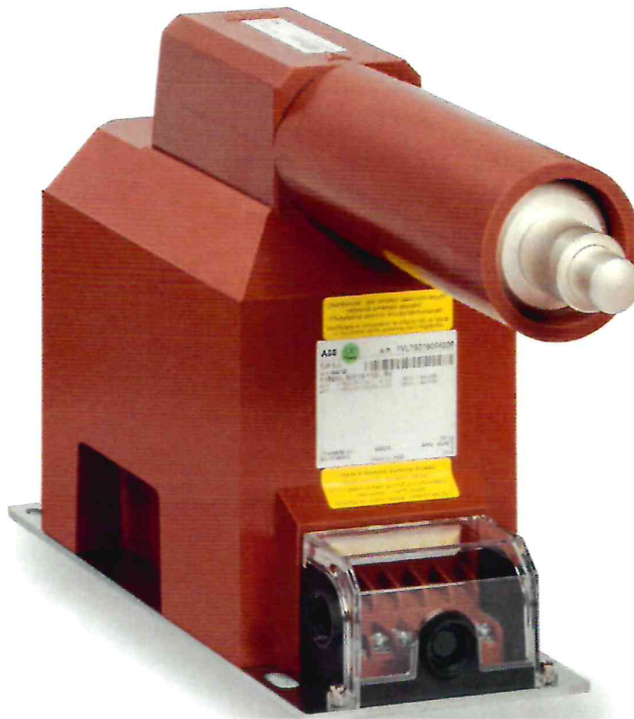
Рисунок 1.1 – Фотография общего вида трансформатора напряжения ТJP 5.1 № 1VLT5209020437
