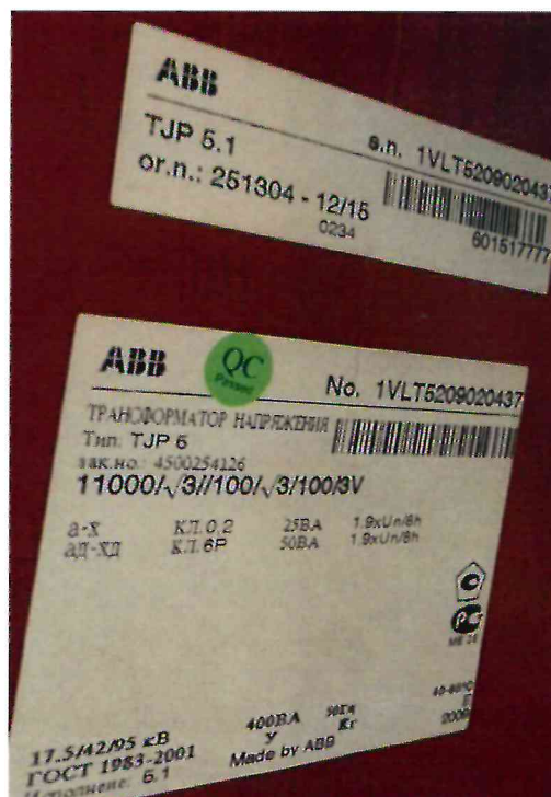
Рисунок 1.2 – Фотография маркировки трансформатора напряжения ТJP 5.1 № 1VLT5209020437
