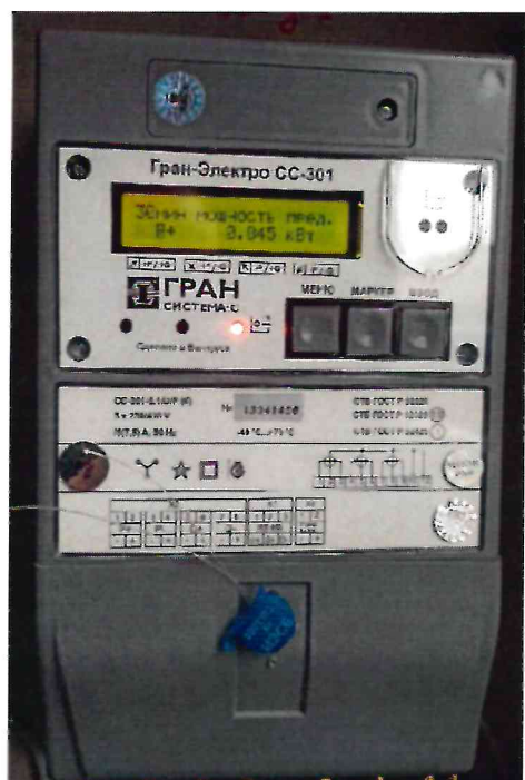
Измерительный канал № 1
