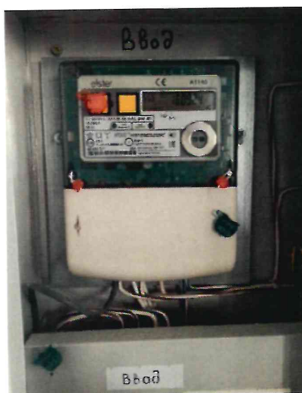
Измерительный канал № 5
