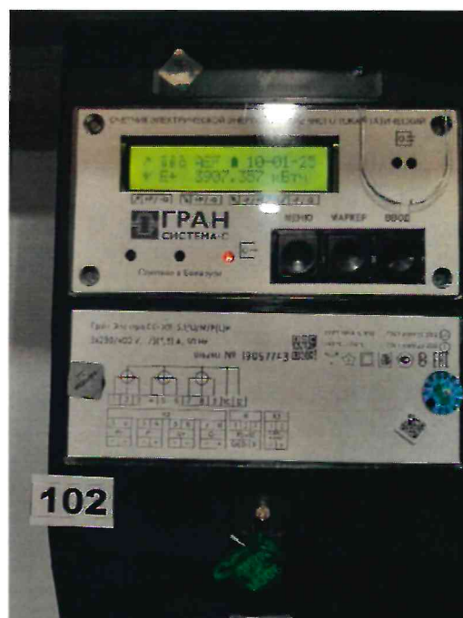
Измерительный канал № 2
