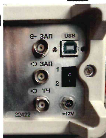
Рисунок 1.1 – Фотографии общего вида и маркировки генераторов ОГ-2-3 (изображения носят иллюстративный характер)
