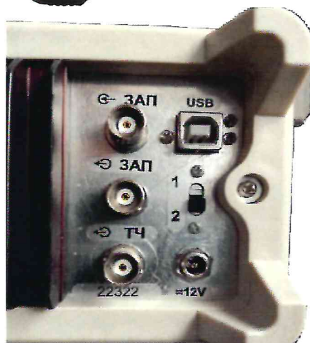
Рисунок 1.1 – Фотографии общего вида и маркировки генераторов ОГ-2-3 (изображения носят иллюстративный характер)
