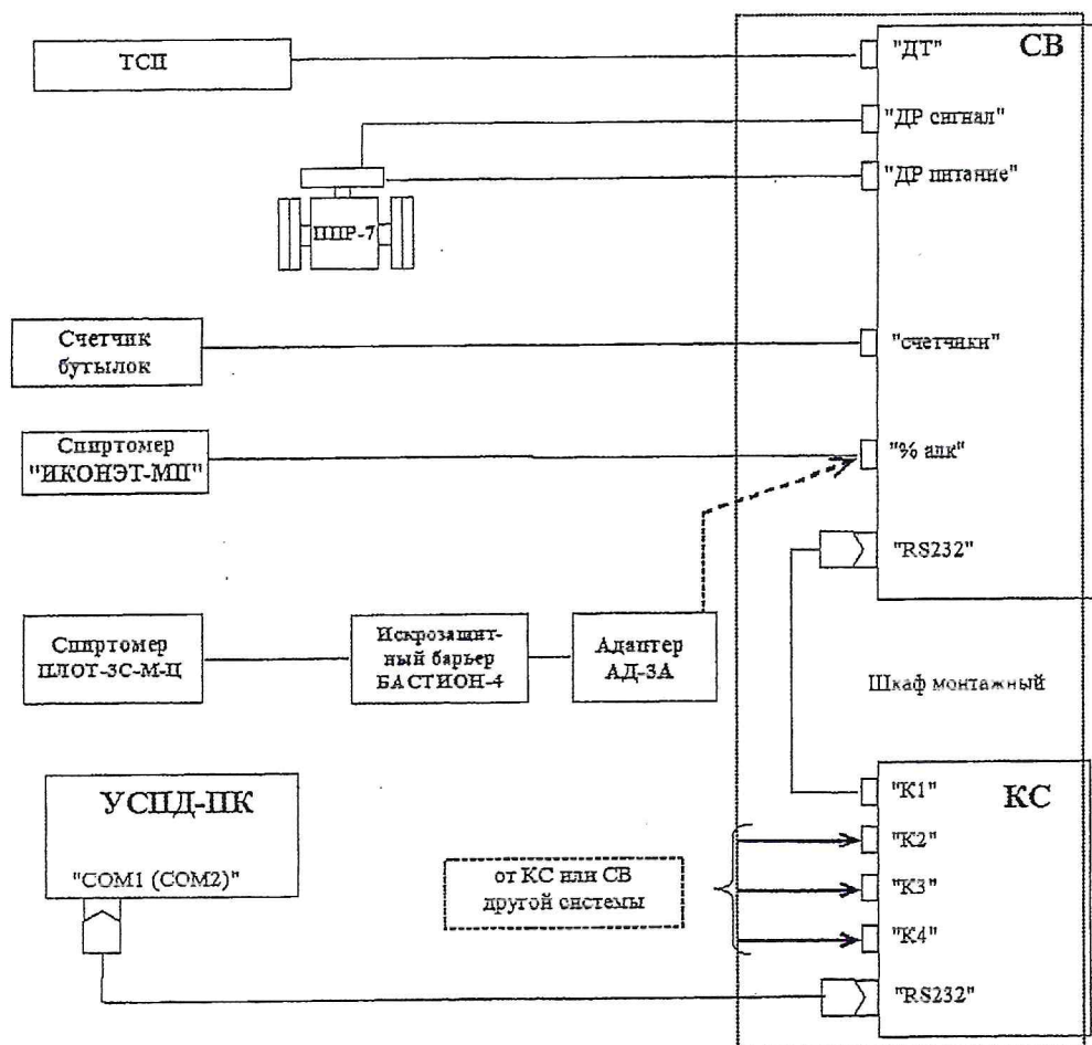
Рисунок 3 – Схема соединений составных частей системы
