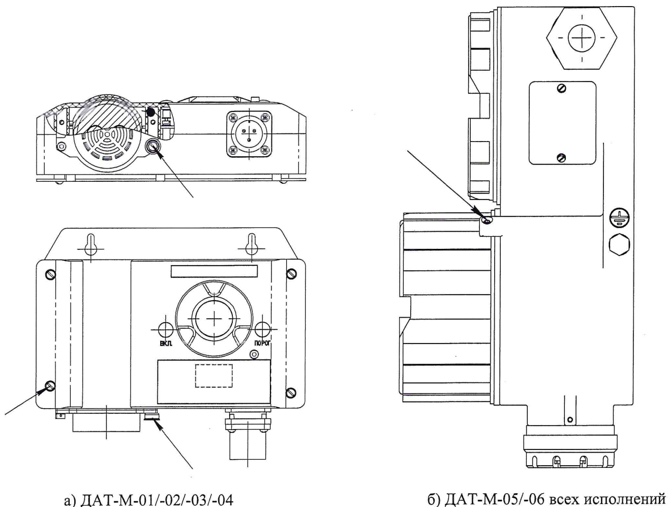
Стрелками указаны места пломбировки от несанкционированного доступа. Рисунок 2 - Схема пломбировки от несанкционированного доступа
