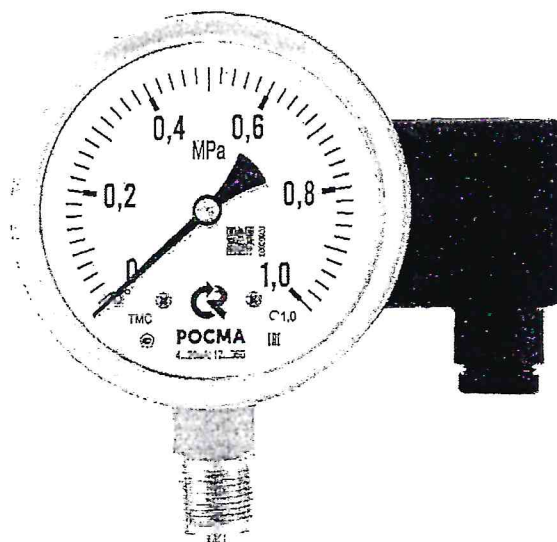
Рисунок 1 – Общий вид приборов
