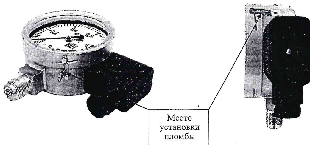
Рисунок 2 - Схема пломбировки манометров от несанкционированного доступа
