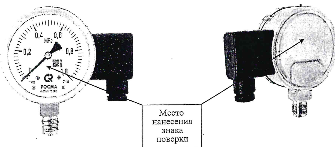
Рисунок 4 – Места нанесения на корпус манометров знака поверки
