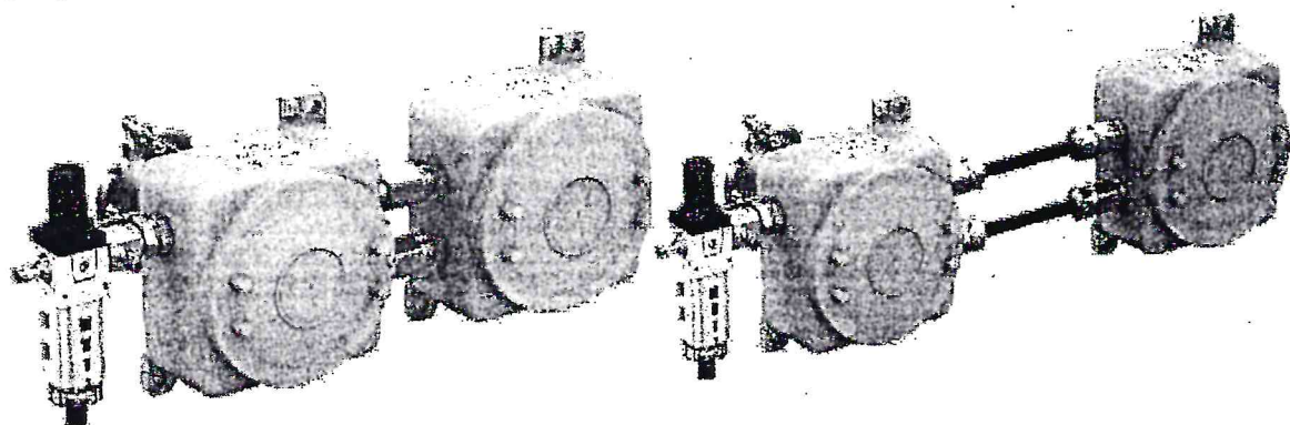
Рисунок 1 – Общий вид измерительного блока газоанализаторов стационарных ЭРИС Оксидиркон 1, слева - жесткое соединение сенсорного и электронного блоков, справа – разделенное
