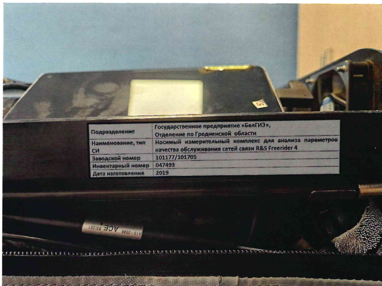
Рисунок 1.2 – Фотография маркировки носимого измерительного комплекса для анализа параметров качества обслуживания сетей связи R&S Freerider 4 № 101177/101705
