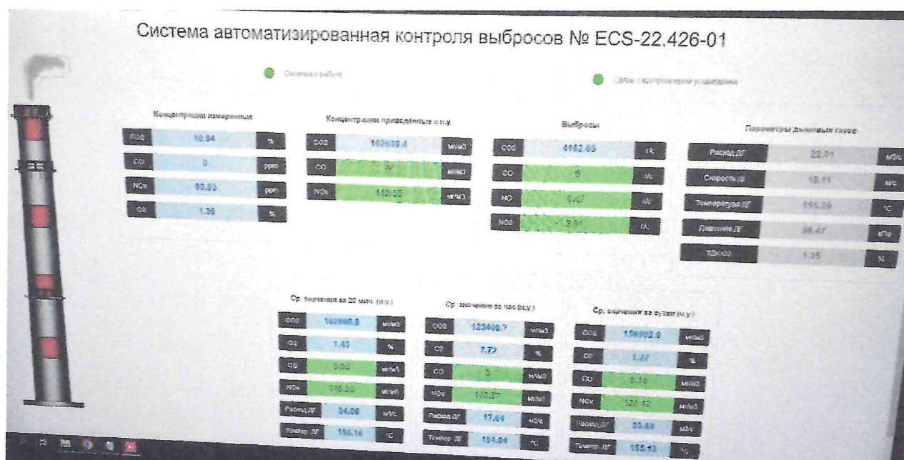
Рисунок 1.7 – Фотография монитора оператора. Система автоматизированная контроля выбросов № ECS-22.426-01
