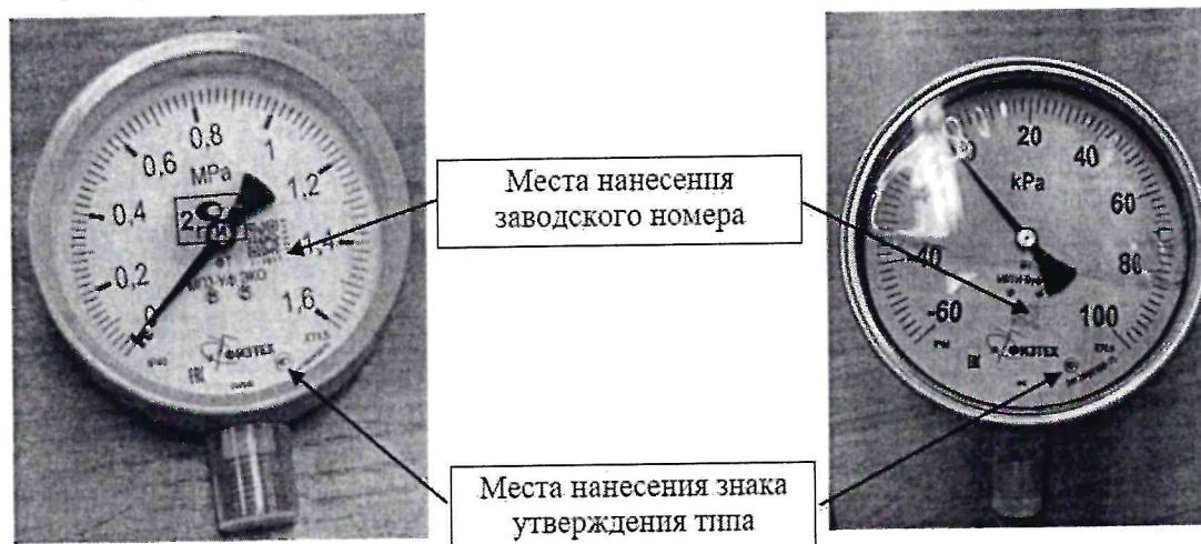
Рисунок 13 – Места нанесения знака утверждения типа и заводского номера
