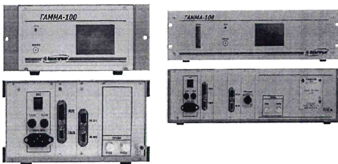
Рисунок 1 - Общий вид газоанализаторов ГАММА-100
