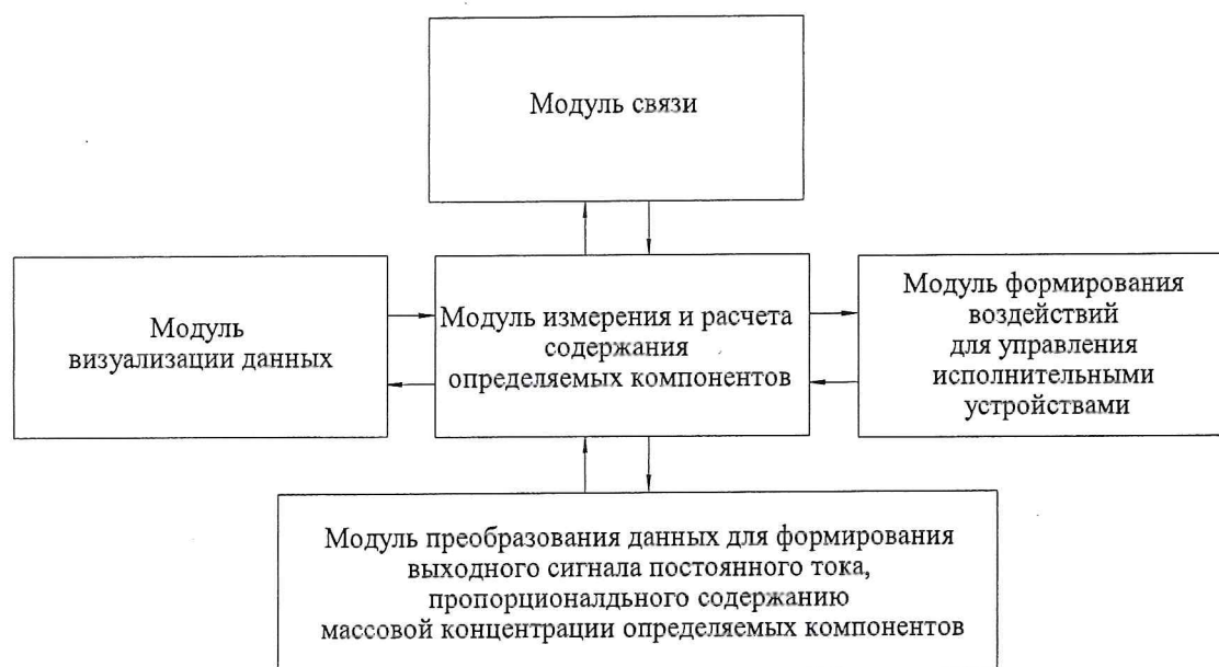
Рисунок 3 - Структура ПО
