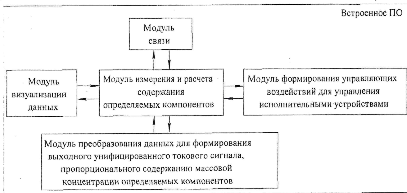
Рисунок 1 - Структура ПО
