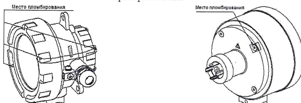
Рисунок 5 – Схема пломбировки ЭКМ от несанкционированного доступа
