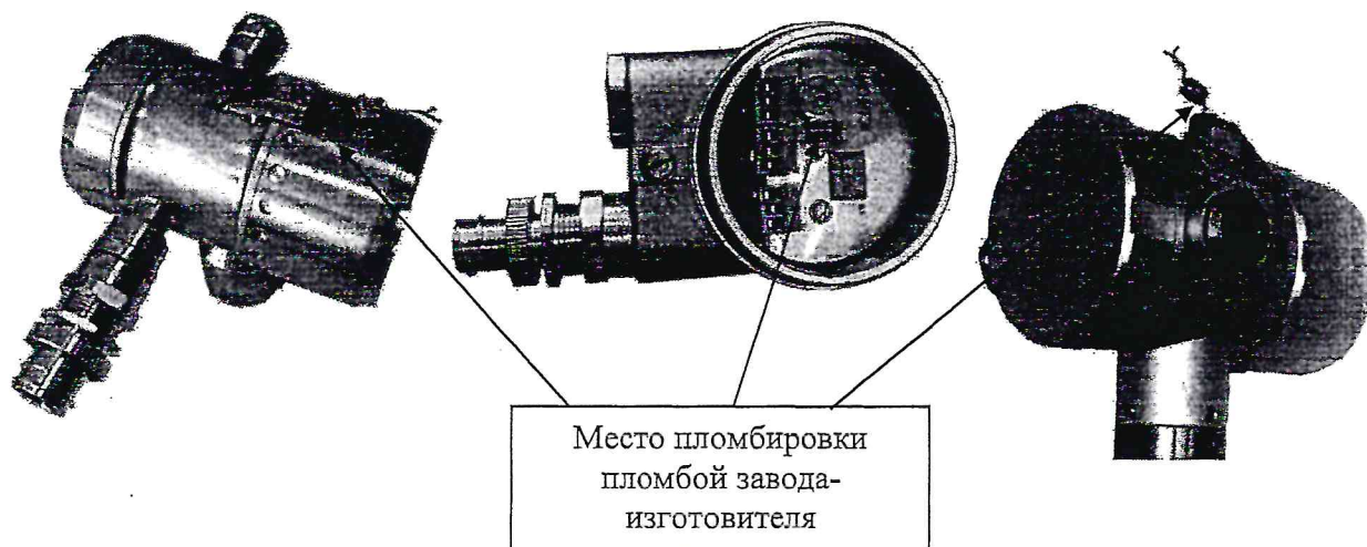
Рисунок 2 – Схема пломбировки электронного блока преобразователя от несанкционированного доступа, обозначение мест пломбировки пломбами завода-изготовителя
