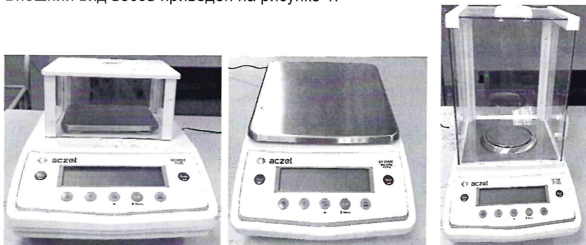
Рисунок 1 – Общий вид весов неавтоматического действия серии СУ.
