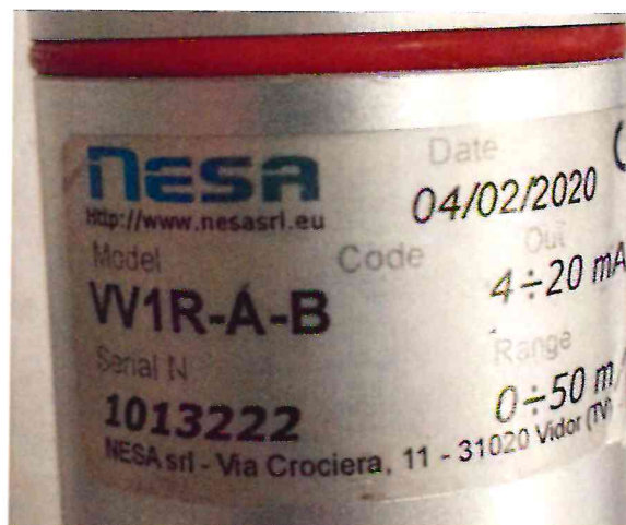
Рисунок 1.2 – Фотография маркировки датчика скорости ветра VV1R № 1013222
