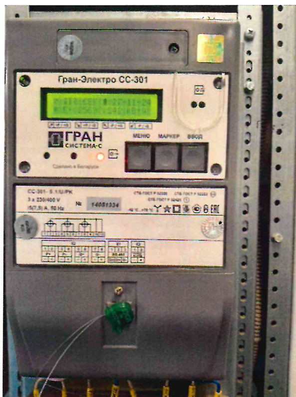
Измерительный канал № 1
