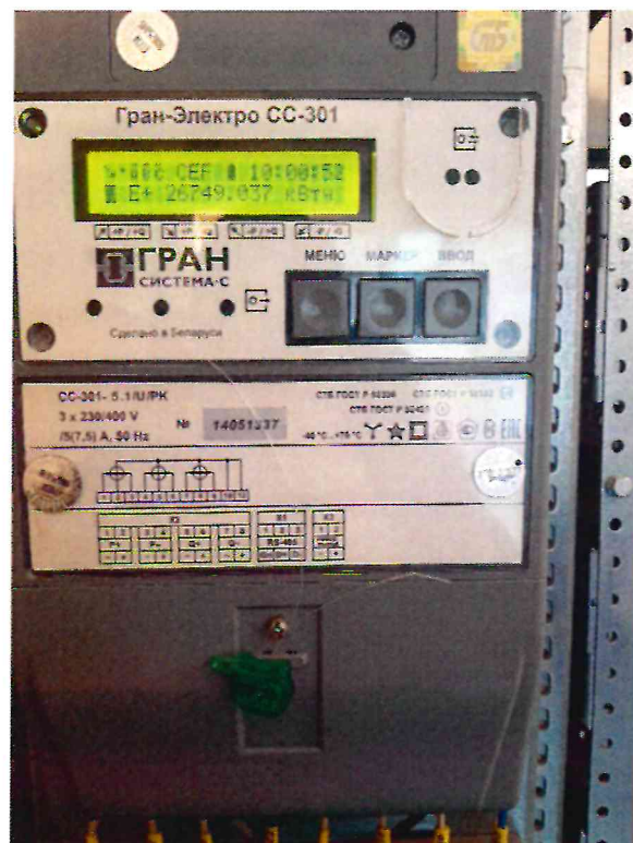
Измерительный канал № 2
