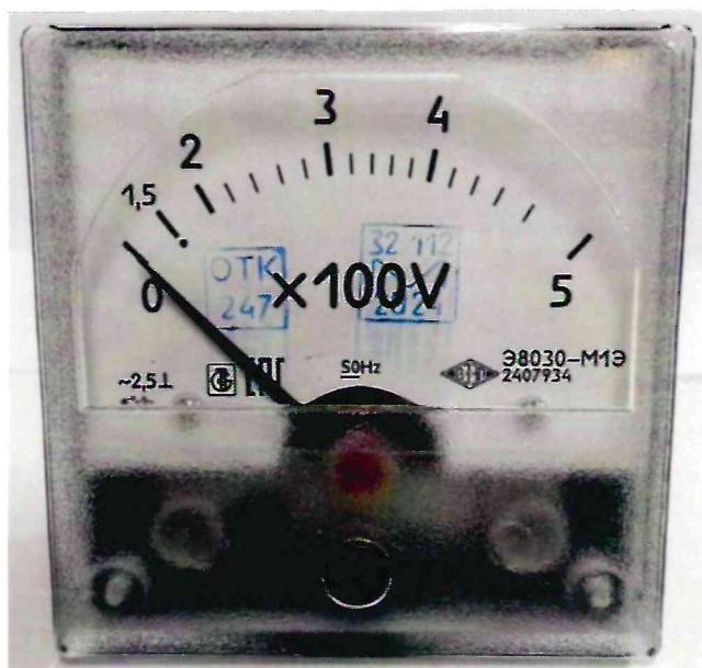
Рисунок 3 - Общий вид вольтметров Э8030-М1Э экспортного исполнения
