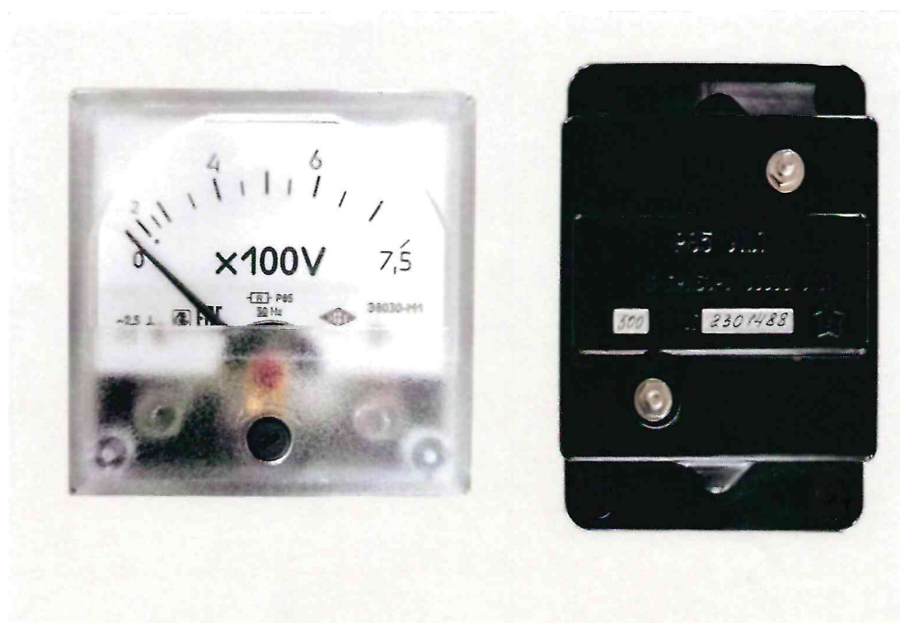
Рисунок 4 - Общий вид вольтметров с индивидуальным добавочным сопротивлением Р85
