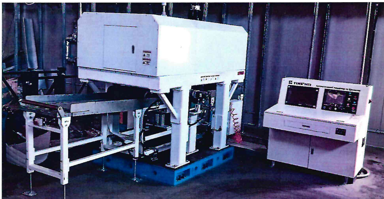
Рисунок 1.1 – Фотография общего вида твердомера автоматического по Бринеллю TIME6479B3 № 038
